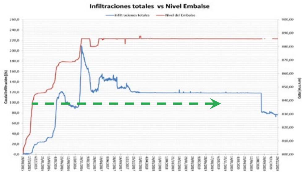
Figura 8. Gráfico Histórico de infiltraciones totales en el Embalse de Bucaramanga.
