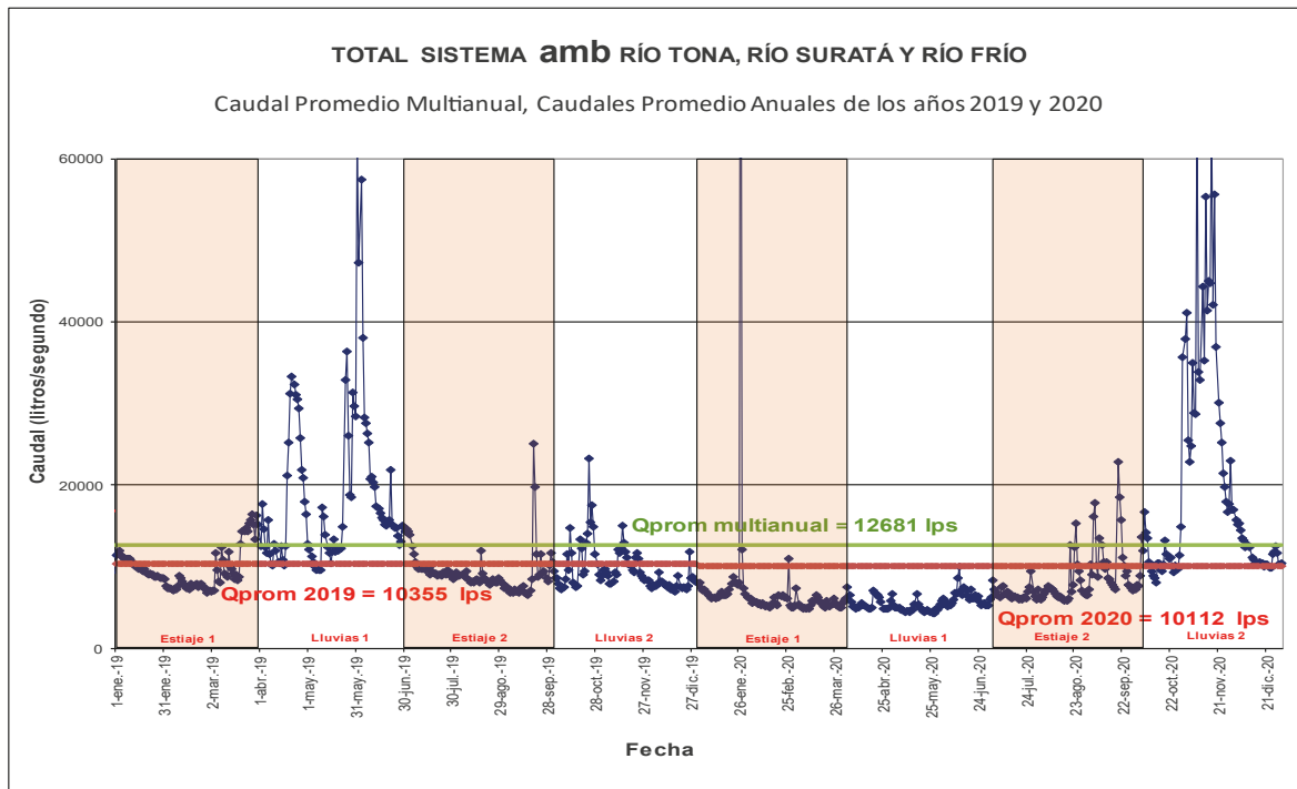
Gráfica DP-01 Caudal Promedio Sistema amb 2020
