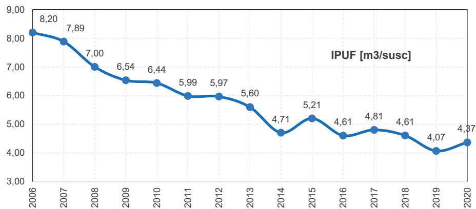
Figura 24. Índice de agua no contabilizada IANC (2006-2020)
