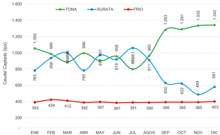
Figura 1. Caudal captado en los sistemas Tona, Frío y Surata
