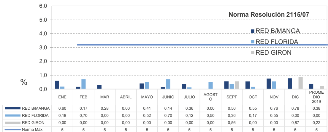
Figura 17. IRCA Promedio mensual del agua en la red de distribución año 2020
