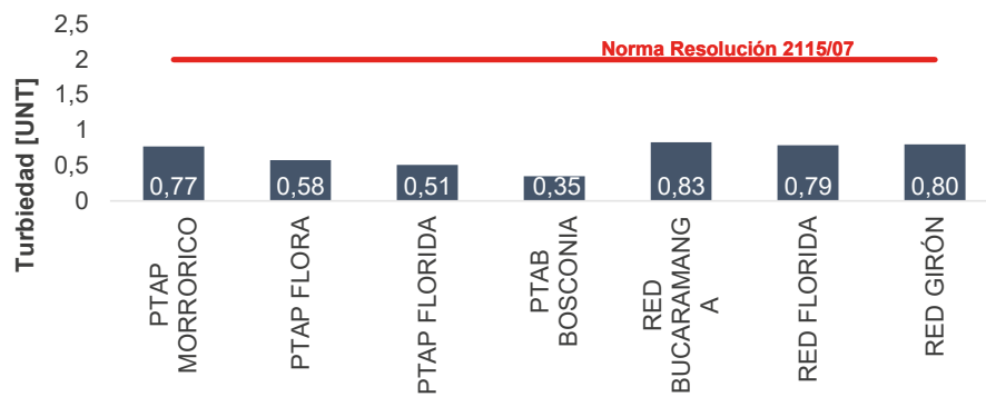
Figura 19. Turbiedad promedio del agua tratada y producida en el año 2020
