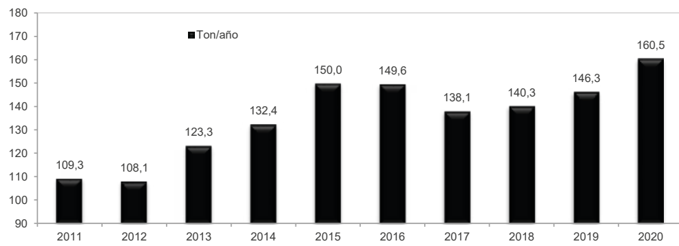
Figura 15. Consumo de Cloro líquido
