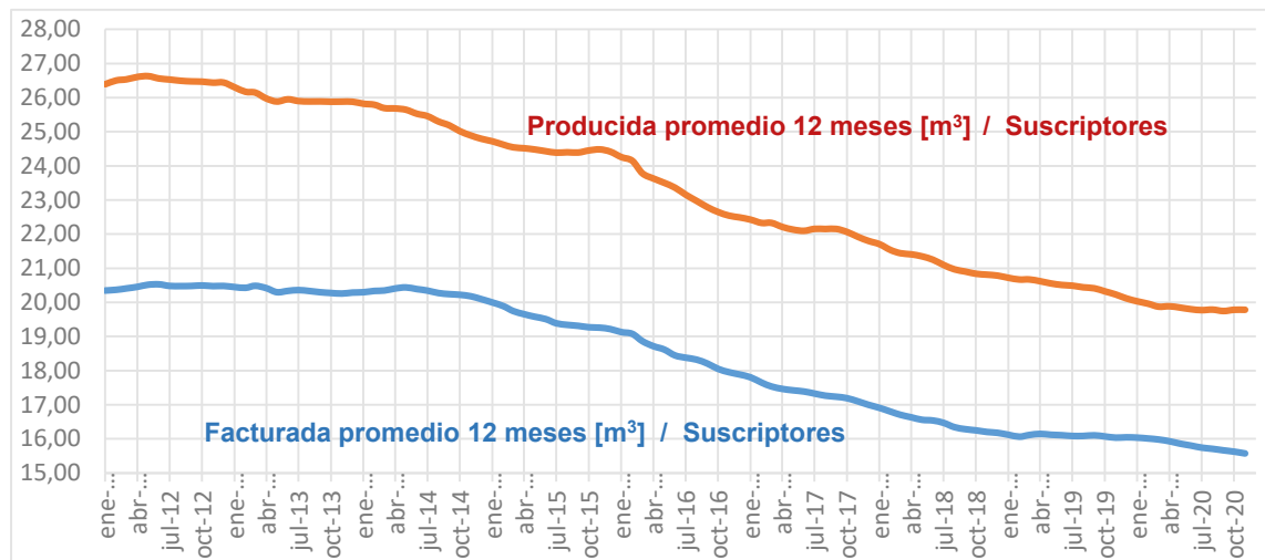
Figura 25. Dotación de agua producida y facturada por suscriptor (2012-2020)
