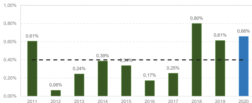
Figura 23. Porcentaje de reposición de redes en el sistema de distribución
