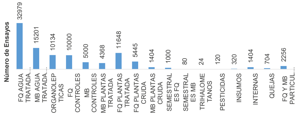
Figura 18. Ensayos de evaluación de la calidad del agua producida y suministrada. Año 2020
