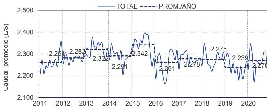
Figura 10. Caudal promedio tratado. Años 2011 a 2019
