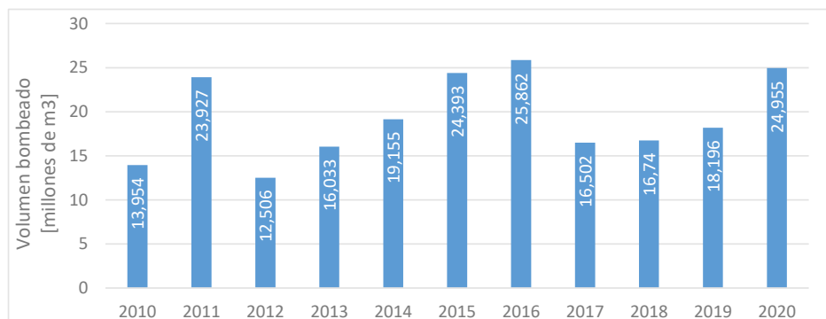
Figura 29. Volumen bombeado por la Estación de Bombeo Bosconia. Años 2010 a 2020
