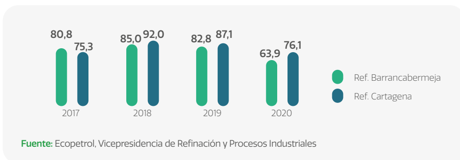
Gráfico 22. Factor de utilización, %
