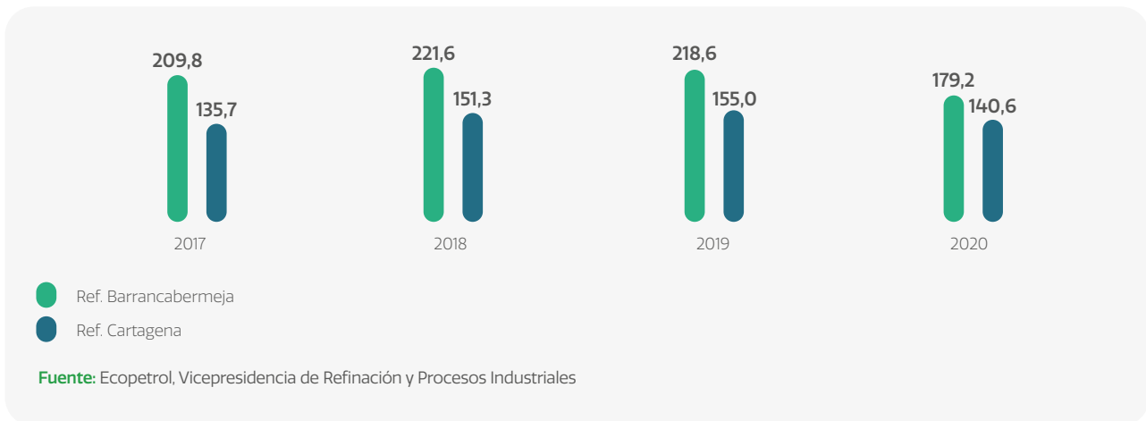
Gráfico 21. Carga de crudo, kbpd
