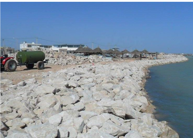
Travaux de protection du littoral - EL Attaya
