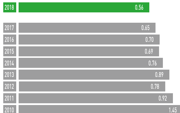
2010-2018 年吨水泥熟料氮氧化物排放量
