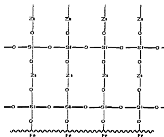
结构示意图
