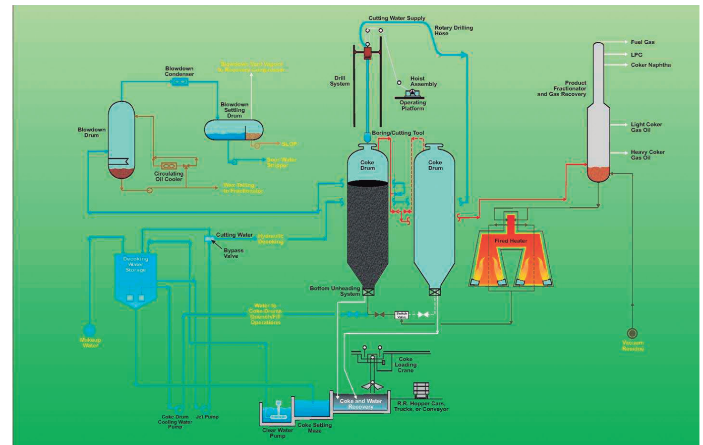
Flujograma de Coquización Retardada de Foster Wheeler
