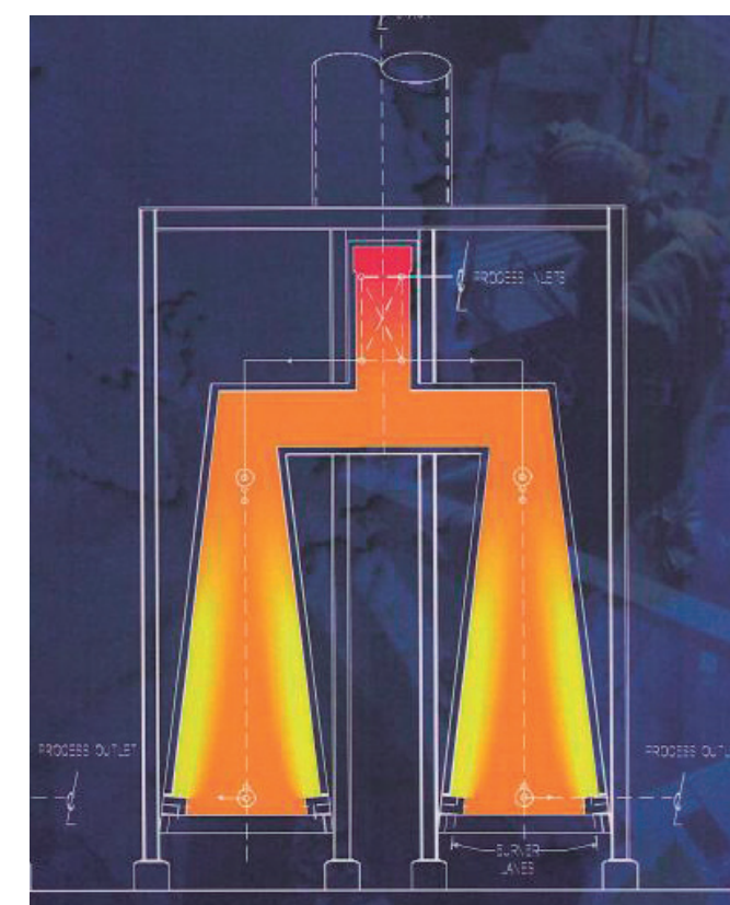
Horno Terrasse Wall de Foster Wheeler
