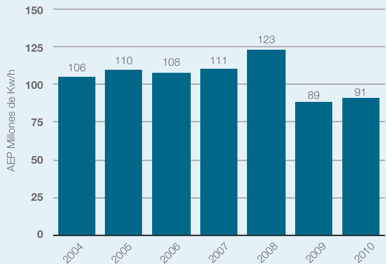
Ahorro de energía primaria (Mill kw/h) en las plantas de cogeneración del Grupo Leche Pascual
