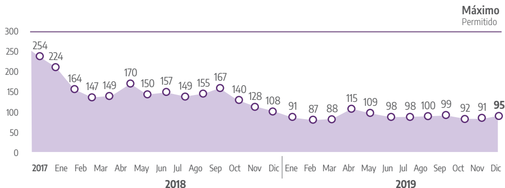
Gráfico 112. Evolución contenido de azufre GASOLINA PROMEDIO NACIONAL PPM
