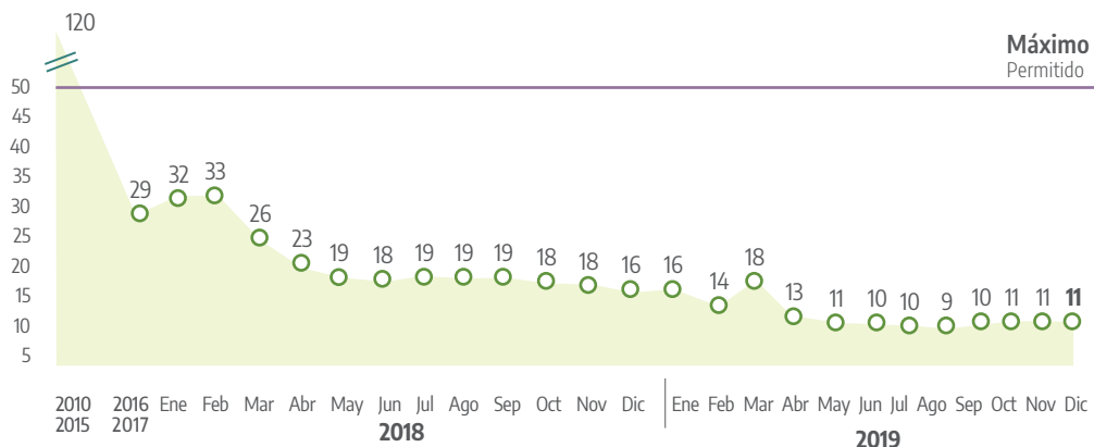
Gráfico 111. Evolución contenido de azufre DIÉSEL B2 PROMEDIO NACIONAL - PPM
