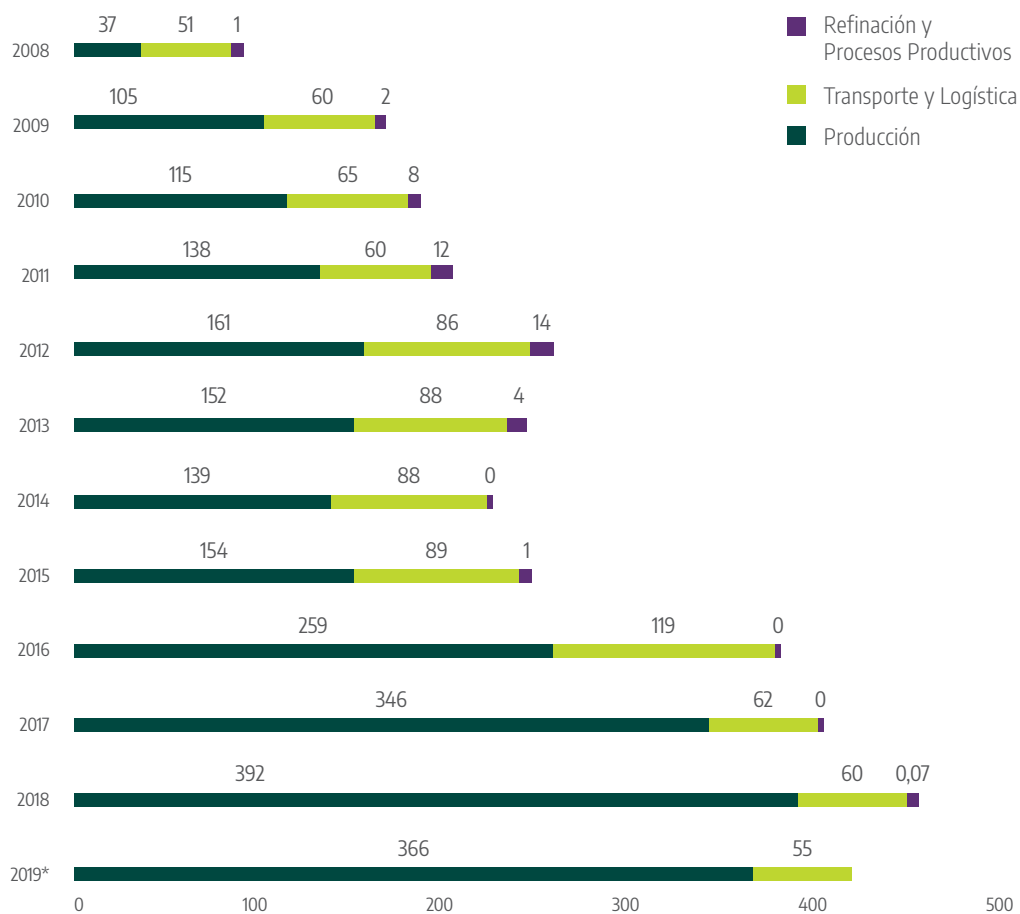
Gráfico 104. Emisiones indirectas anuales por procesos operativos (Kilotoneladas CO 2 e)
