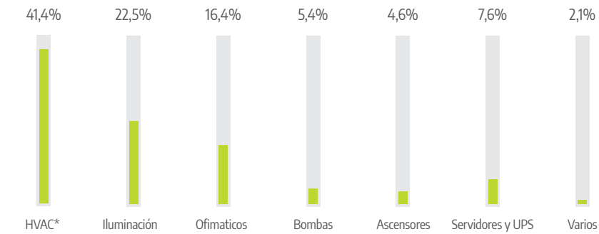
Gráfico 115. Distribución del consumo de energía Edificio Teusacá - 2019
