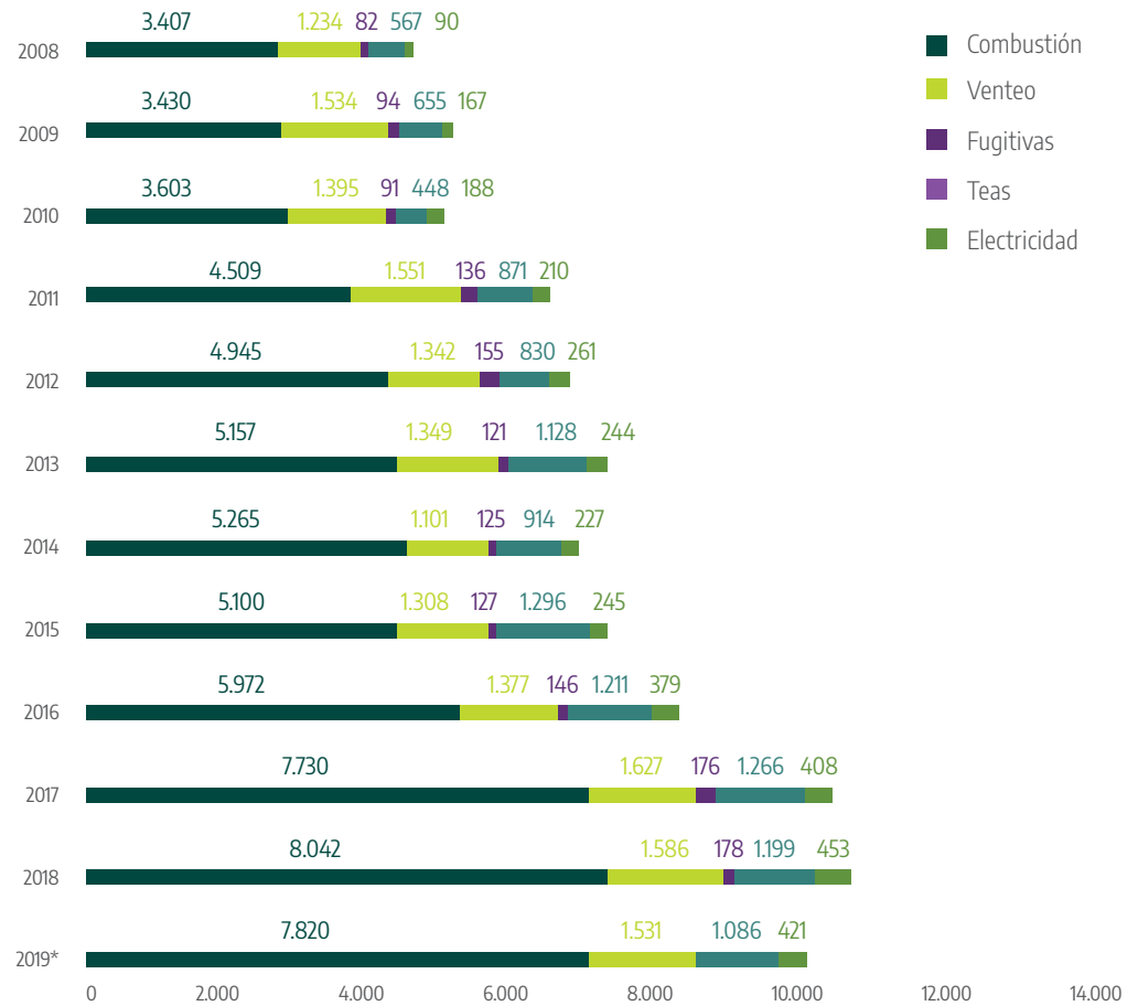
Gráfico 102. Emisiones totales de GEI por tipo de fuente (kilotoneladas CO 2 e)
